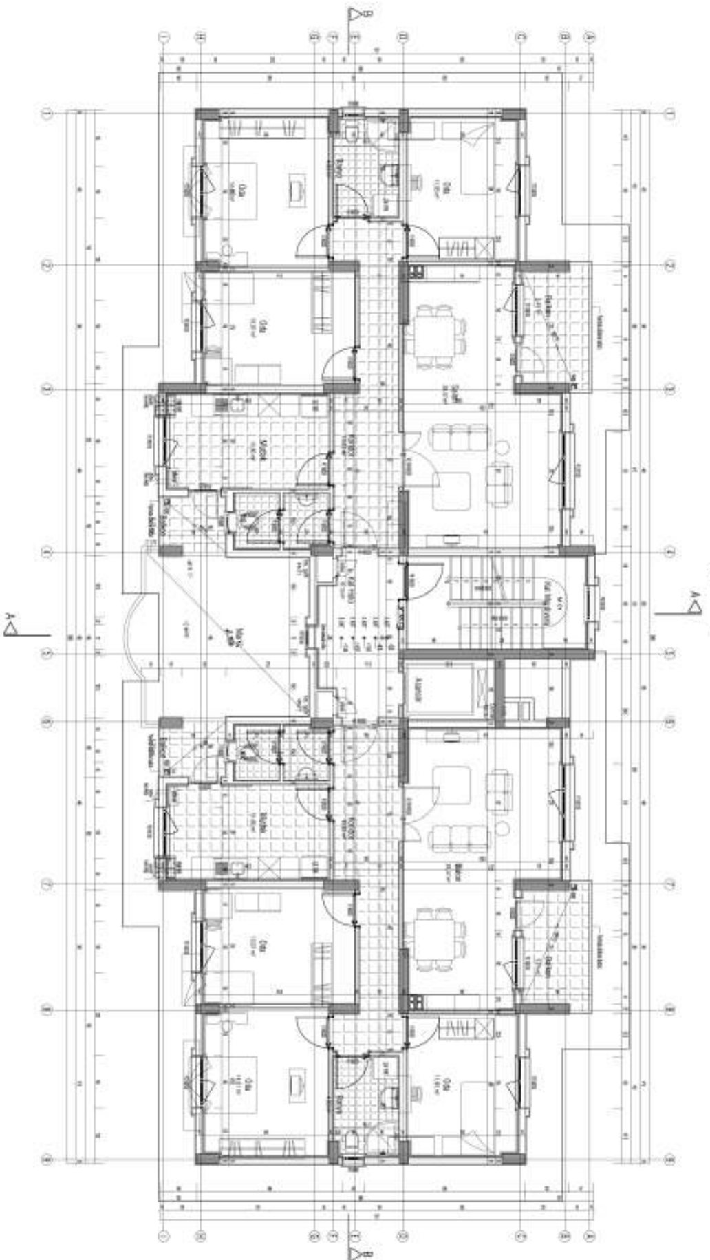
TİPİK KAT PLANI
